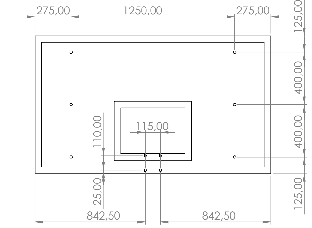
Schema di foratura per fissaggio tabellone e canestro Drilling template for fixing the backboard and basket
