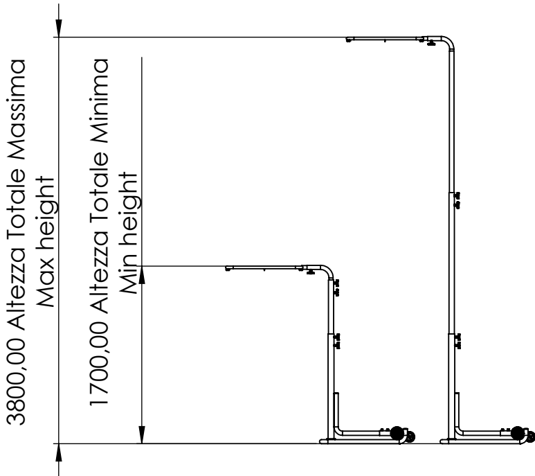
Altezze comprensive di basamento (non incluso) Heights including basement (not included)
